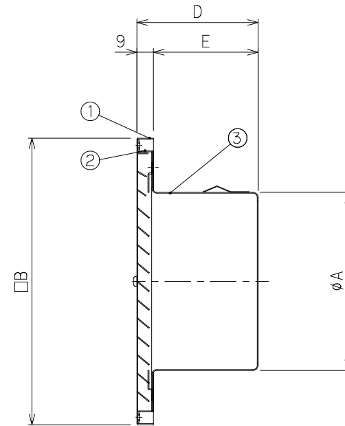
A-A断面
