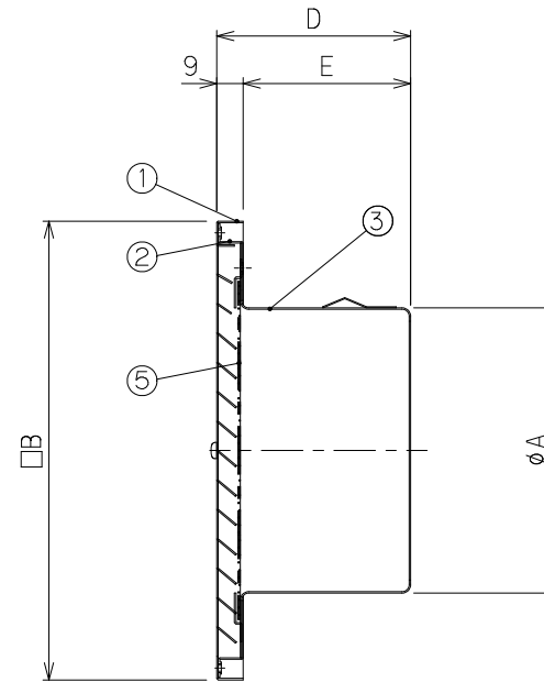
A-A断面
