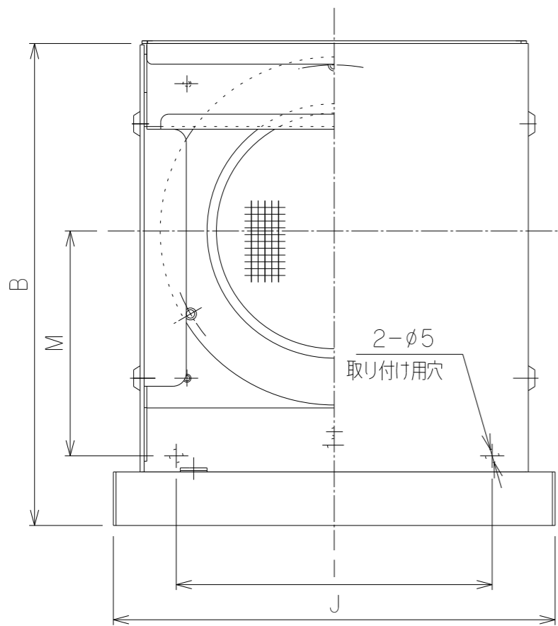
A-A矢視図
